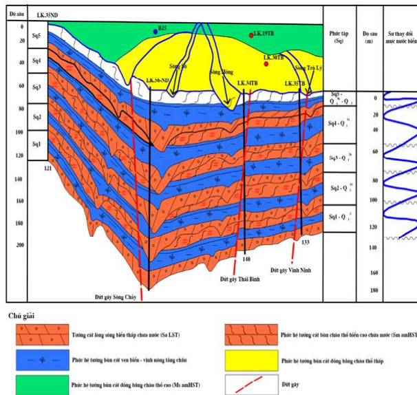
Hình 5. Sơ đồ khối mặt cắt tương trầm tích và vị trí các tầng chứa nước và cách nước theo 5 phức tập liên kết [16] có bổ sung và chỉnh sửa mới
