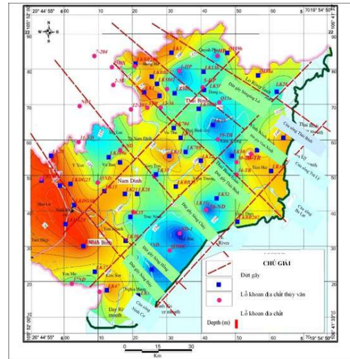
Hình 2. Bản đồ cấu trúc địa chất Hệ Tứ và đứt gãy khu vực hạ lưu châu thổ Sông Hồng (Phùng Văn Phách và nnk, 2007; Trần Nghi có bổ sung sửa chữa, 2022)
