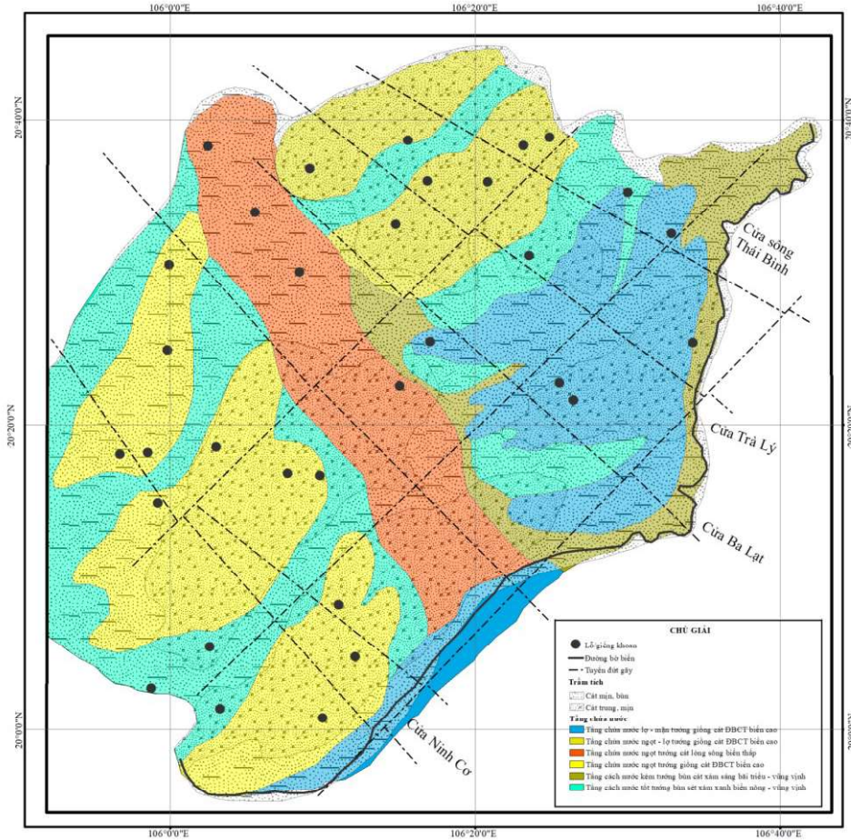
Hình 7. Bản đồ phân vùng mặn nhạt theo tương trầm tích khu vực Thái Bình và Nam Định [[16]] có bổ sung và chỉnh sửa mới
