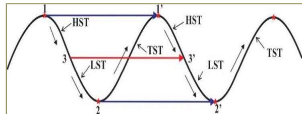
Hình 4. Mô hình địa tầng phân tậ của Trần Nghi (2017)
