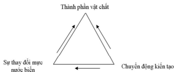
Hình 3. Mối quan hệ nhân-quả giữa thành phần trầm tích-sự thay đổi mực nước biển và chuyển động kiến tạo (Trần Nghi, 2002)
